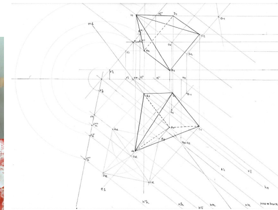
Pedro, 11ºAno, Geometria Descritiva
